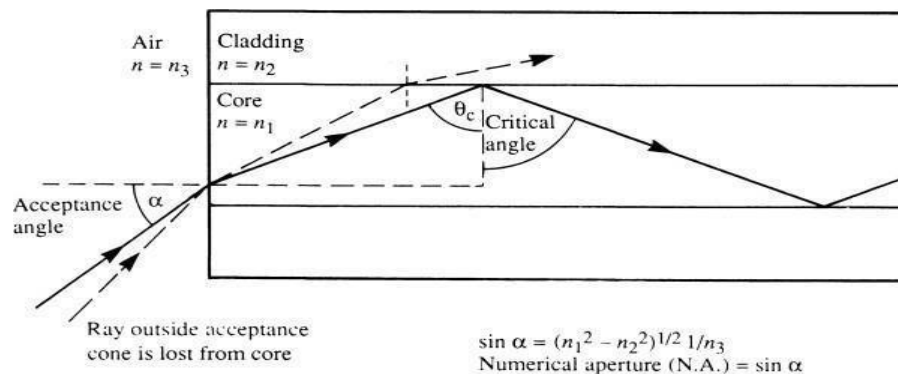
Fig. 3.7 Refraction
