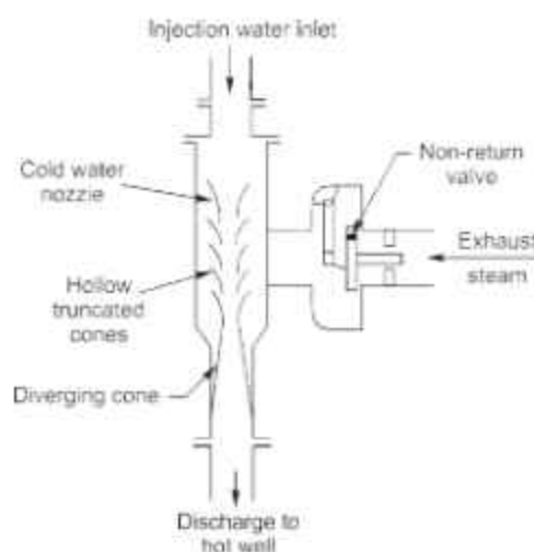
Fig. 1.22. Ejector Condenser
