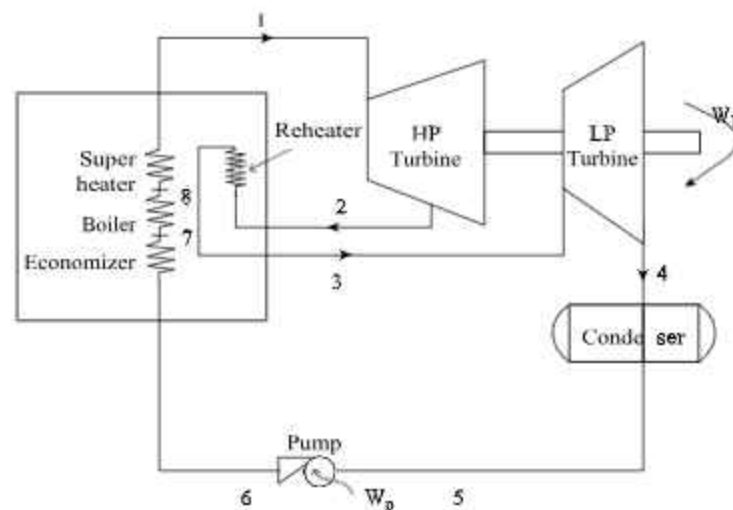
Fig. 4.17 Reheat
