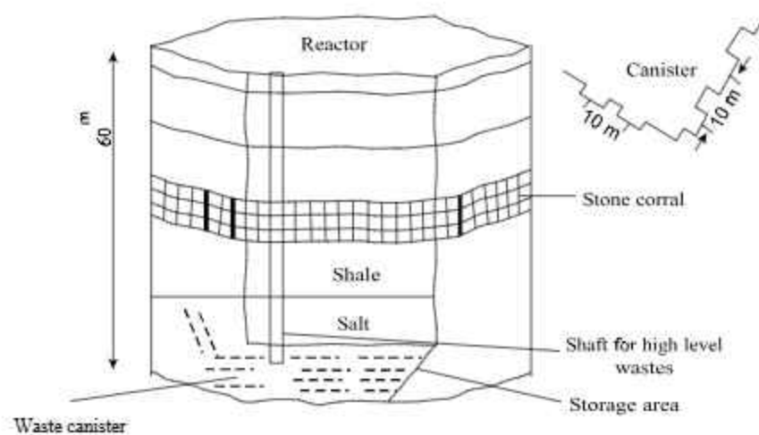
Fig. 16.34 Disposal of LLW
