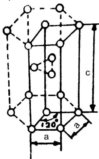
EX ----Be,Tc,Zn
